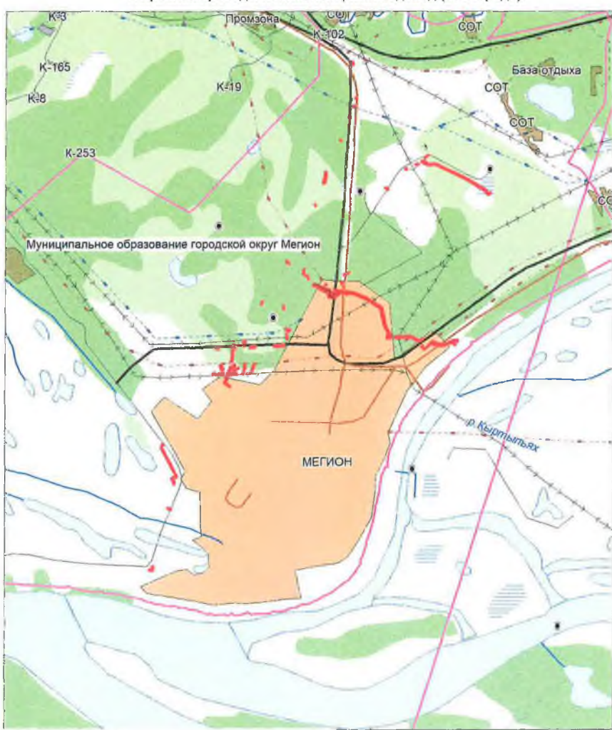
Карта-схема испрашиваемого земельного участка под объект: «Обустройство Ватинского месторождения нефти. Нефтегазопроводы и низконапорный водовод (VI очередь)»
