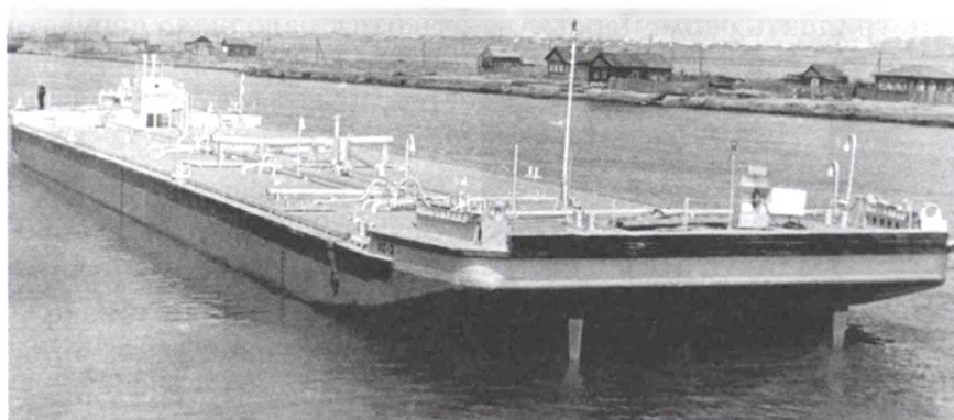
Нефтеналивная баржа проекта 459 Н
