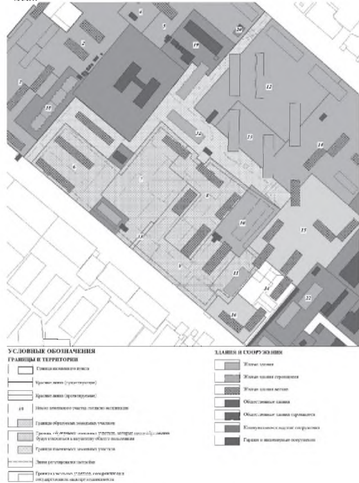
ПРОЕКТ ВНЕСЕНИЯ ИЗМЕНЕНИЙ В ПРОЕКТ ПЛАНИРОВКИ И ПРОЕКТ МЕЖЕВАНИЯ ТЕРРИТОРИИ 5 МИКРОРАЙОНА Г. МЕГИОНА ЧЕРТЕЖ МЕЖЕВАНИЯ ТЕРРИТОРИИ М 1:1500
