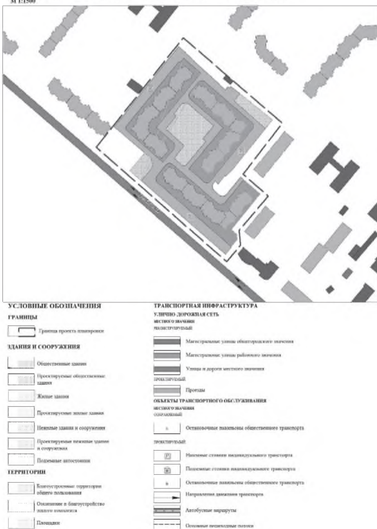
ПРОЕКТ ВНЕСЕНИЯ ИЗМЕНЕНИЙ В ПРОЕКТ ПЛАНИРОВКИ И ПРОЕКТ МЕЖЕВАНИЯ ТЕРРИТОРИИ 5 МИКРОРАЙОНА Г. МЕГИОНА СХЕМА ОРГАНИЗАЦИИ УЛЧНО-ДОРОЖНОЙ СЕТИ И СХЕМА ДВИЖЕНИЯ ТРАНСПОРТА М 1:1500
